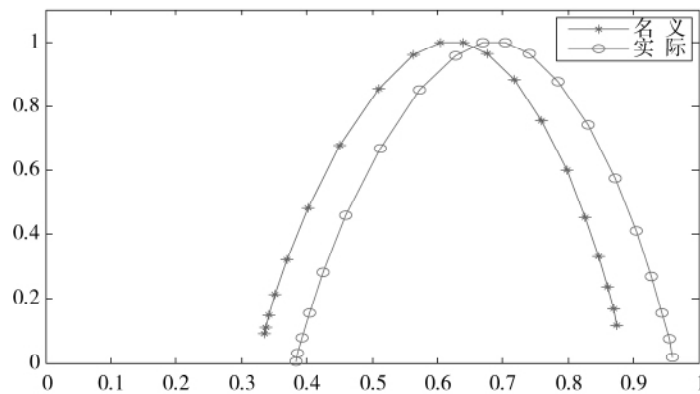
图6 复旦人民币汇率指数收益率序列的多重分形谱图
