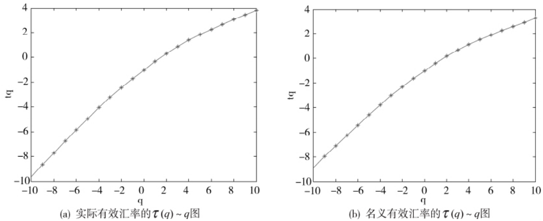
图5 复旦人民币汇率收益率序列的质量指数图
