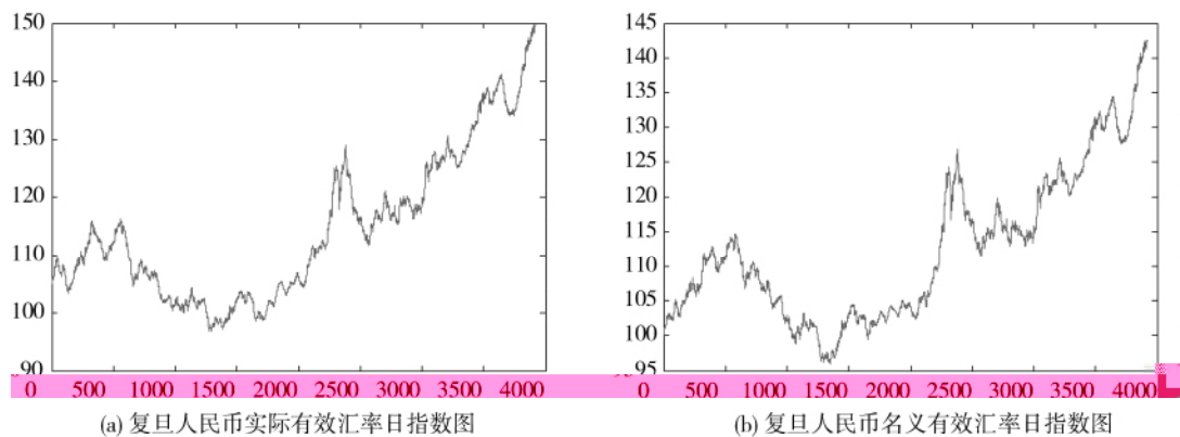
图1 复旦人民币有效汇率指数序列的波动图
