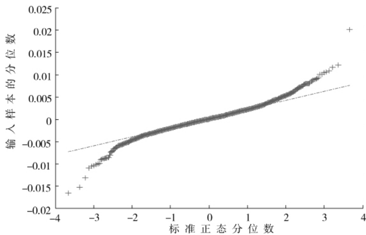
图7 复旦人民币实际有效汇率收益率序列的Q-Q分位图
