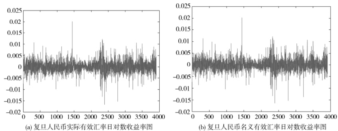
图2 复旦人民币有效汇率指数的日对数收益率图
