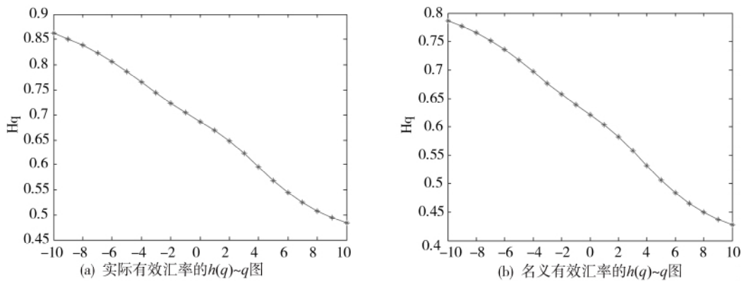
图4 复旦人民币汇率收益率序列的广义 Hurst 指数图
