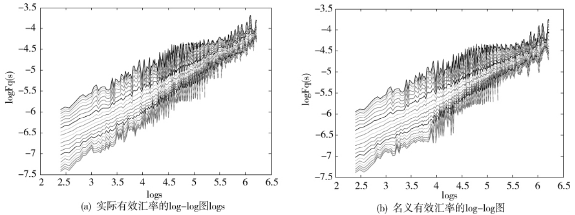
图3 复旦人民币汇率收益率序列波动函数的 log-log 图
