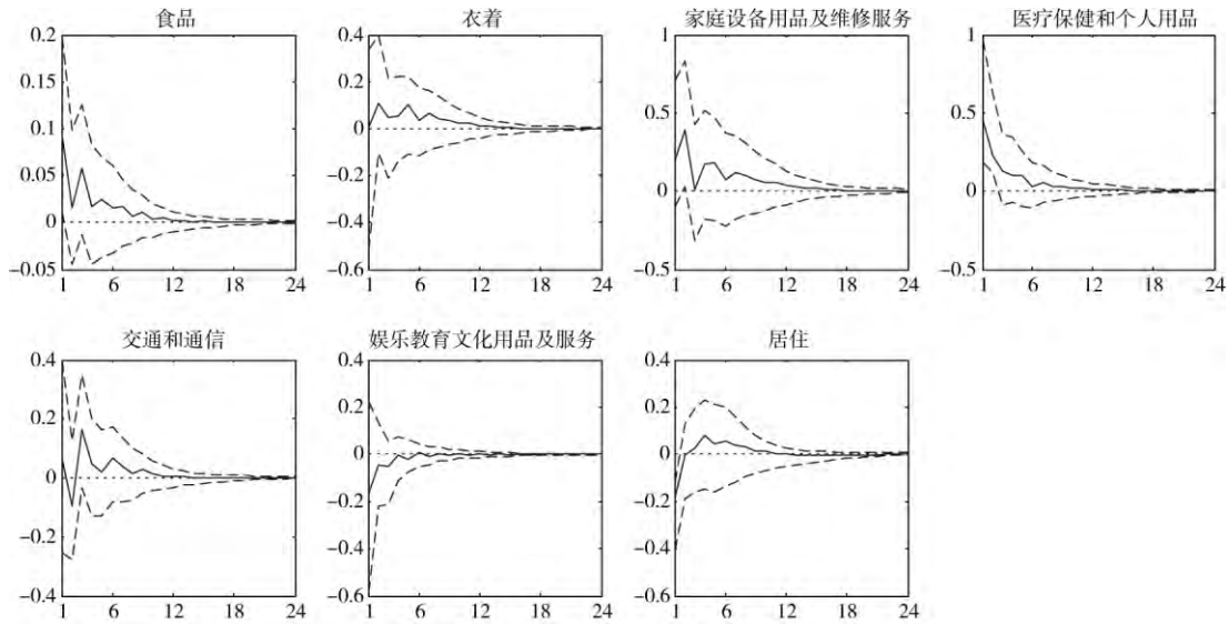
图5 CPI分项数据的冲击响应
