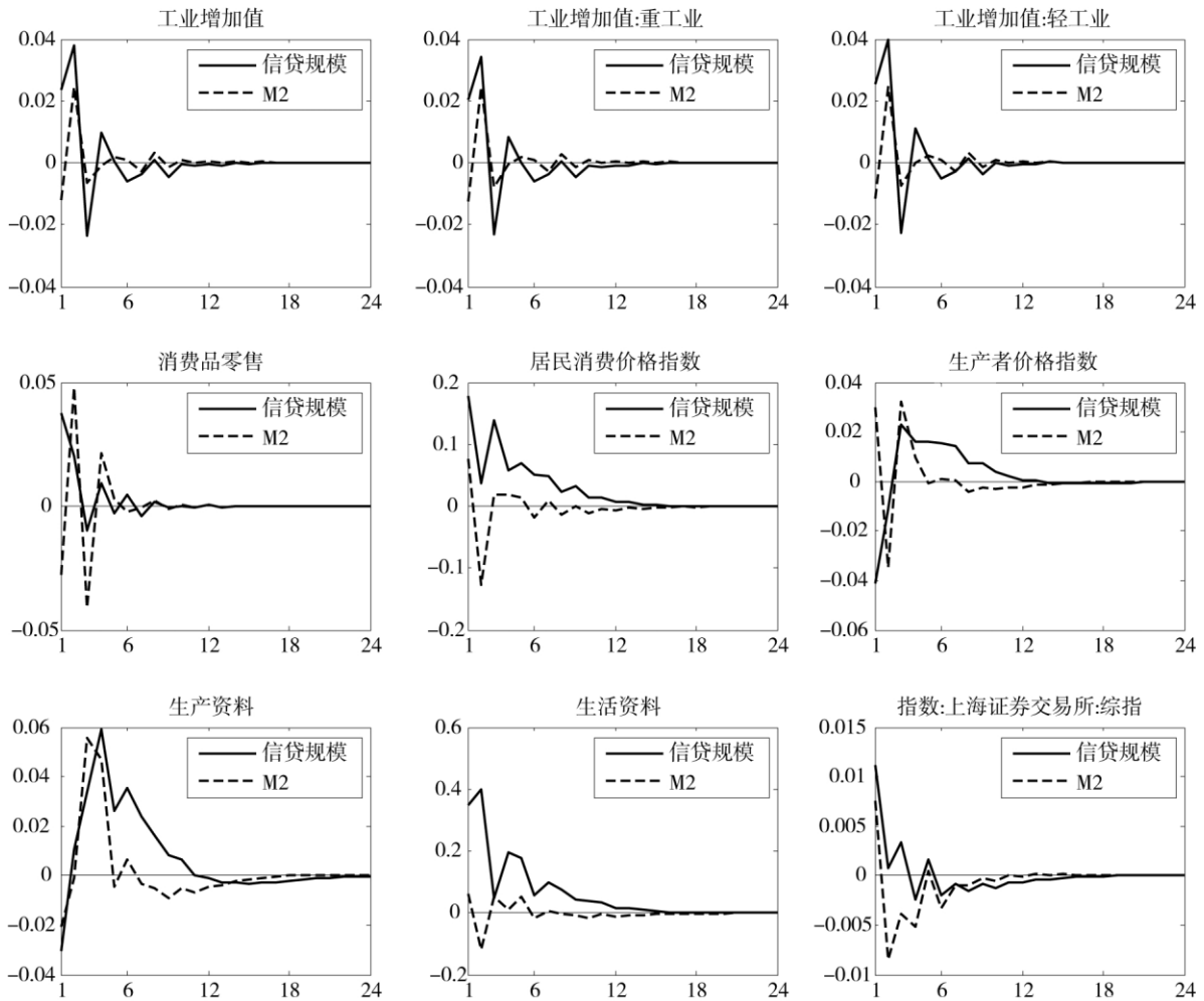
图1 重要总体经济指标对信贷量和货币量的冲击响应
