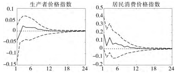
图 2 PPI 和 CPI 的冲击响应
