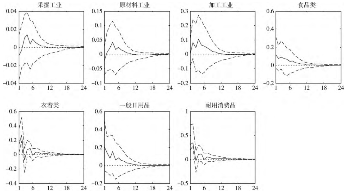
图 4 PPI 中生产资料和生活资料部分分项数据的冲击响应
