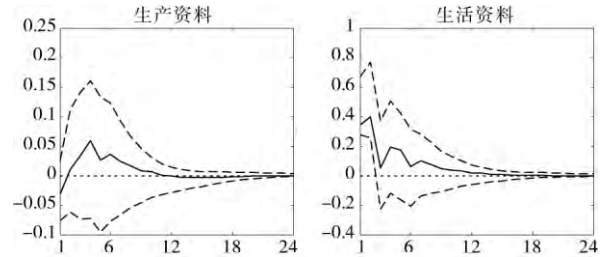
图 3 PPI 中生产资料部分和生活资料部分的冲击响应
